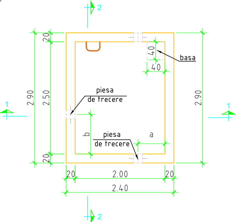
SECTIUNE ORIZONTALA SCARA 1:50
