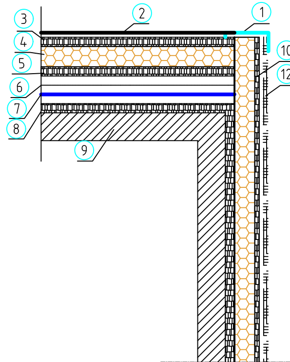
Detali- invelitoare,trotuar
