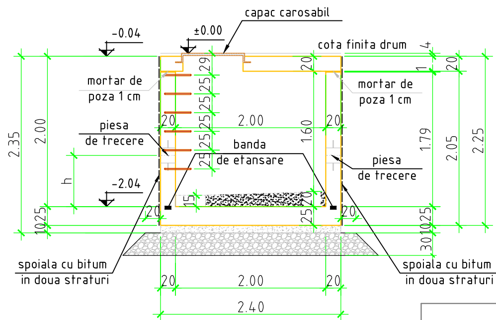
SECTIUNEA 2-2 SCARA 1:50
