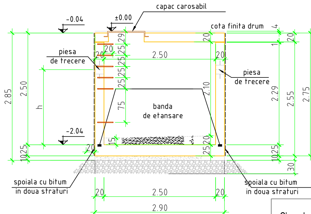
SCARA 1:50
