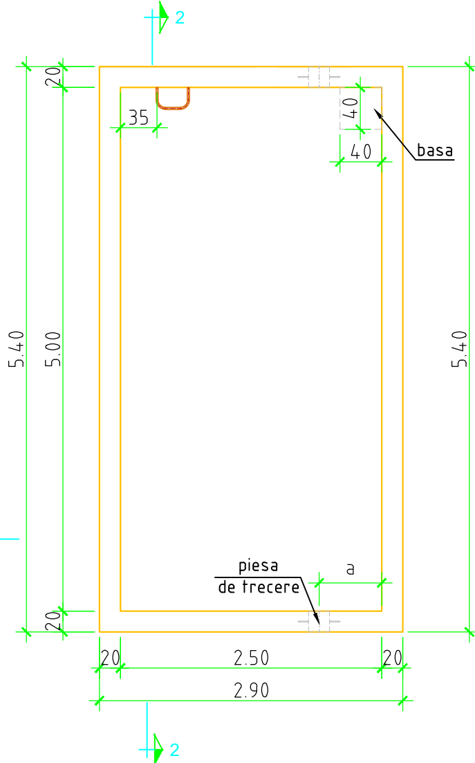
SECTIONE ORIZONTALA SCARA 1:50
