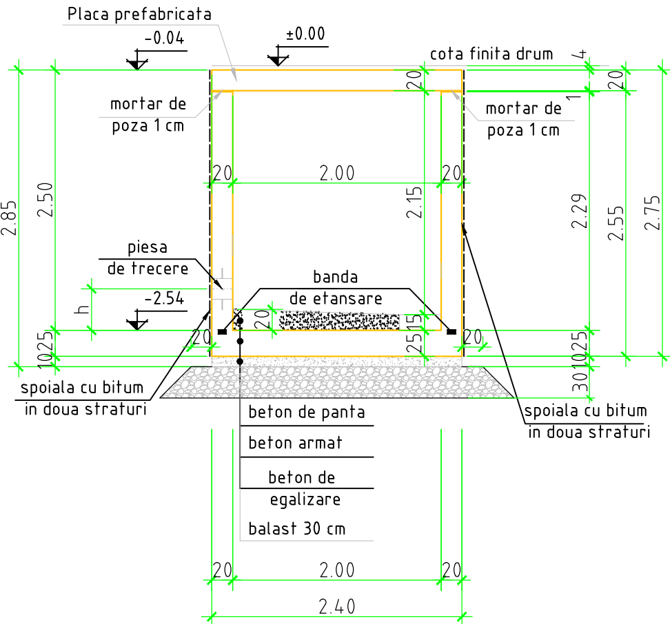
SECTIUNEA 1-1 SCARA 1:50
