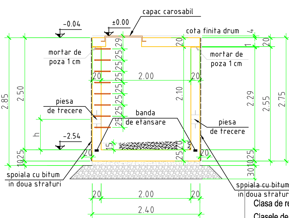
SECTIUNEA 2-2 SCARA 1:50
