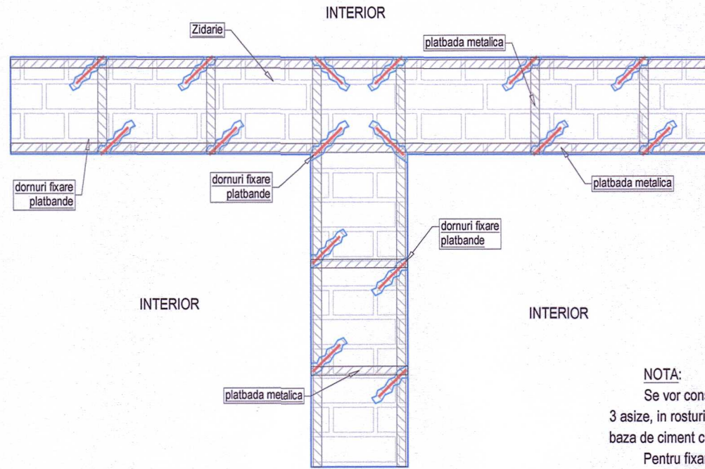
Detaliu dispunere platbade metalice la intersecții de pereti / elevatii
