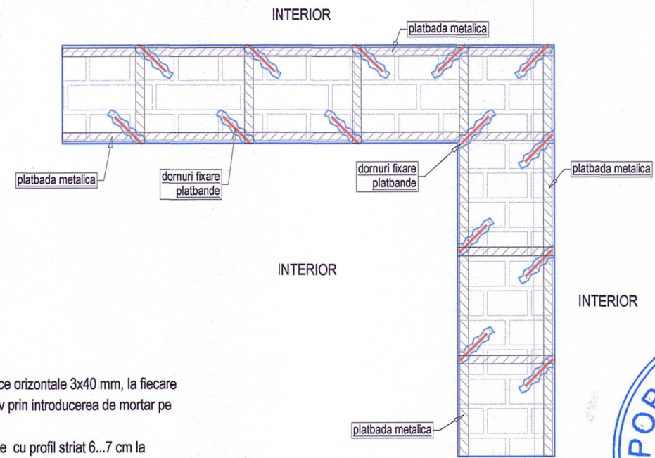
Detaliu dispunere platbade metalice la intersecții de pereti / elevatii
