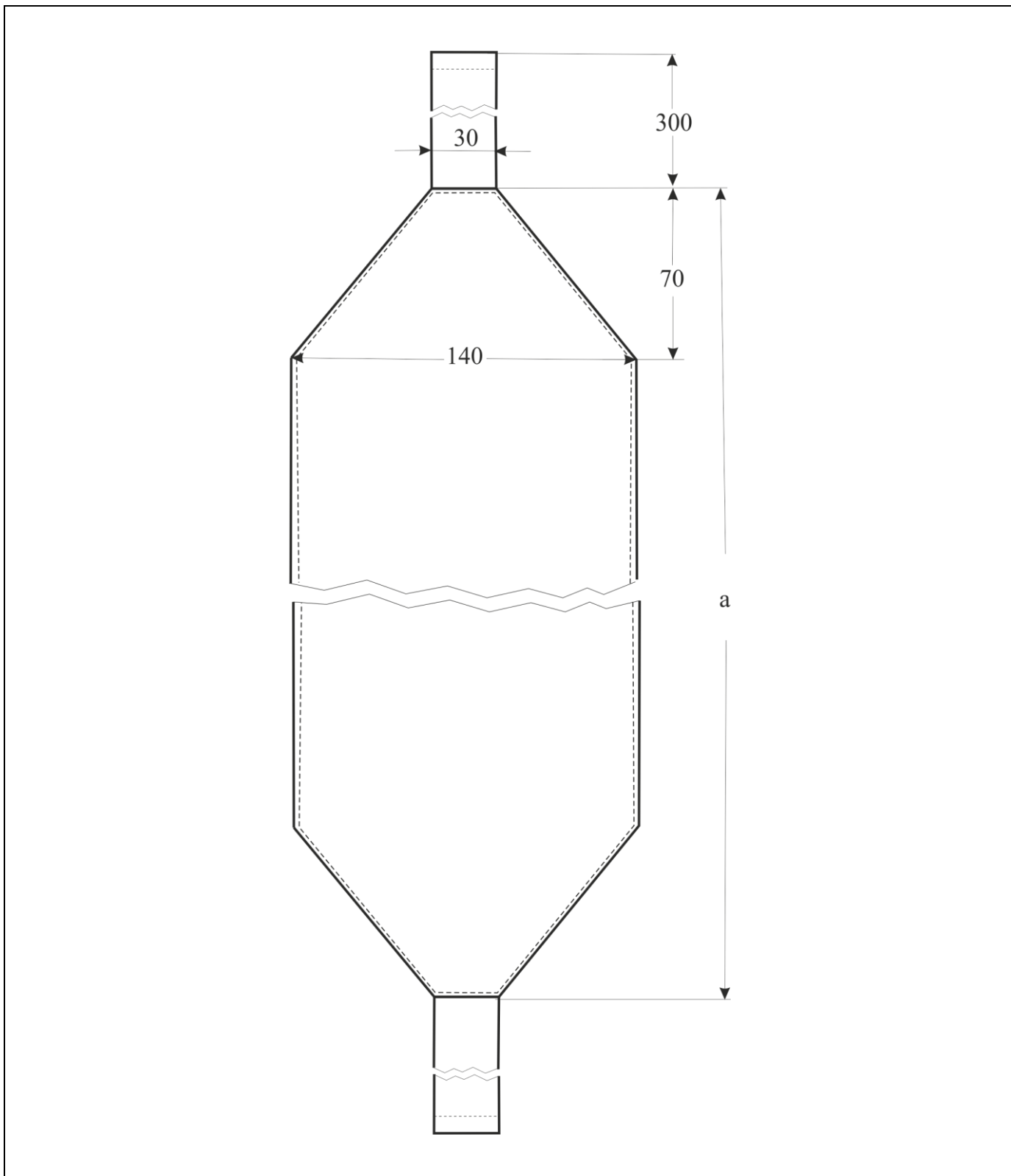
DESENUL NR. 1 – Prezentare generală/cote în mm
