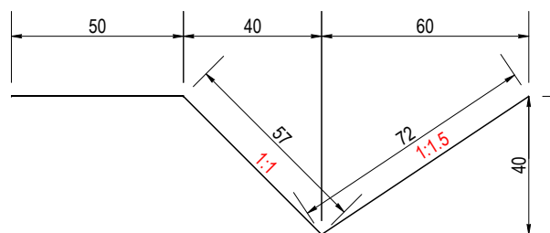
Detaliu șanț tip P1
