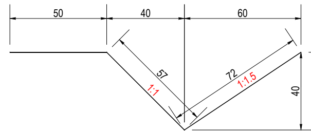
Detaliu șant tip P1 Sc. 1:20
