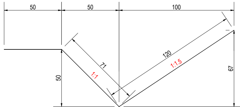
Detaliu șanț tip P2 Sc. 1:20
