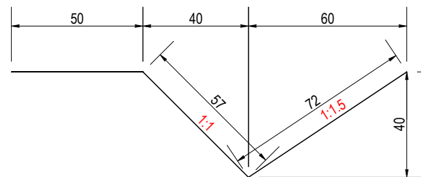
Detaliu șanț tip P1 Sc. 1:20
