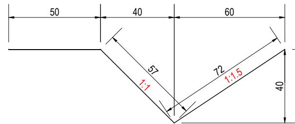
Detaliu șanț tip P1
