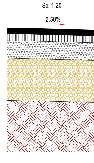
Detaliu sistem rutier Sc. 1:20
