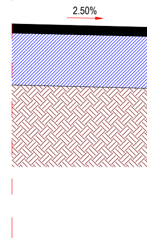
Detaliu sistem rutier
