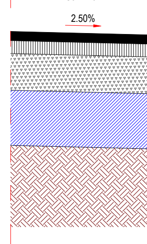
Detaliu sistem rutier Sc. 1:20
