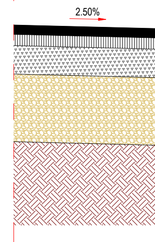
Detaliu sistem rutier Sc. 1:20
