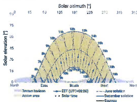
(Diagrama elevatie-azimut)
