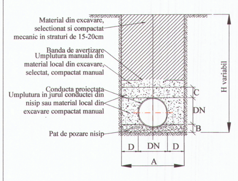
DETALIU SAPATURA PENTRU REțele DE APA SI CANALIZARE
