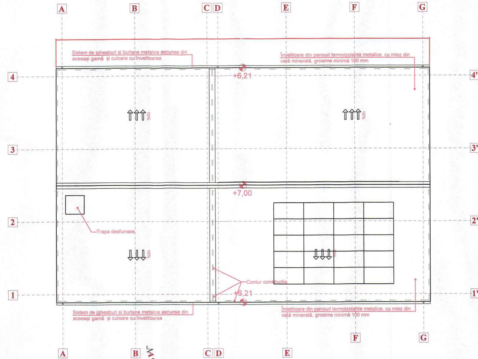
PLAN ÎNVELITOARE
