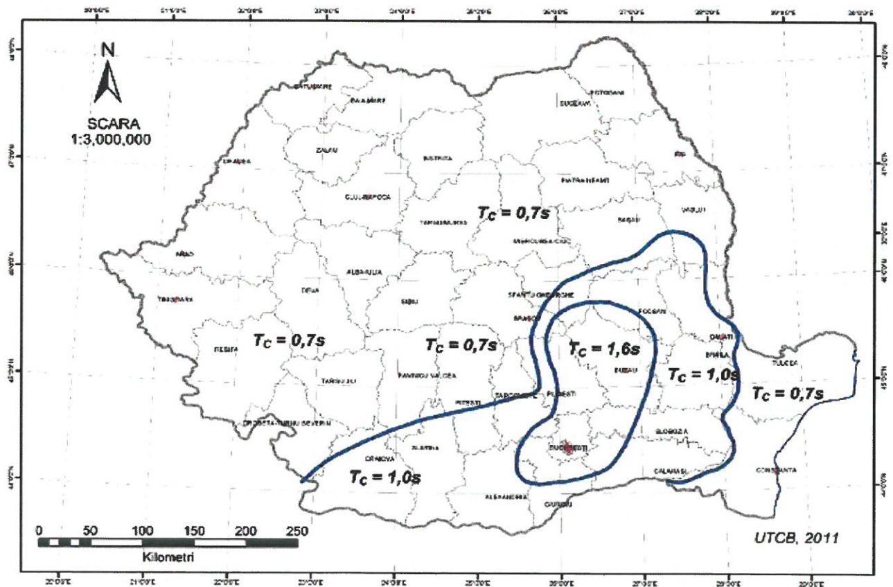
Figura 3. Zonarea în termeni de perioada de control (colt) T_c a spectrului de răspuns.
