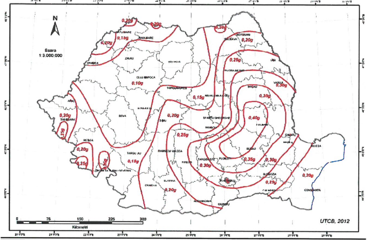
Figura 21. Zonarea valorilor de vârf ale accelerației terenului pentru proiectare a_g cu IMR = 225 ani și 20% probabilitate de depășire în 50 de ani.
