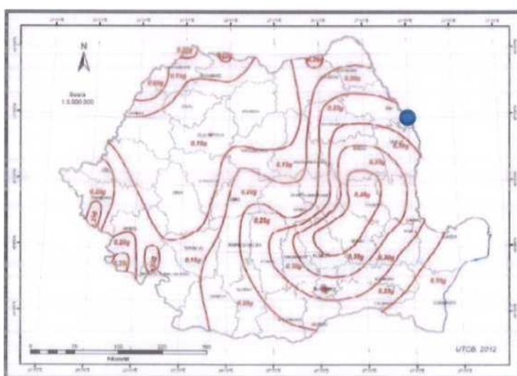
Figura 1. Zonarea valorii de vârf a accelerației terenului pentru proiectare cutremure având IMR 225 de ani și probabilitate de depășire de 20% în 50 de ani
