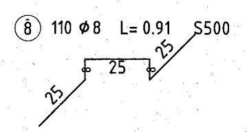
Detaliu capre 2buc/mp Scara 1:25
