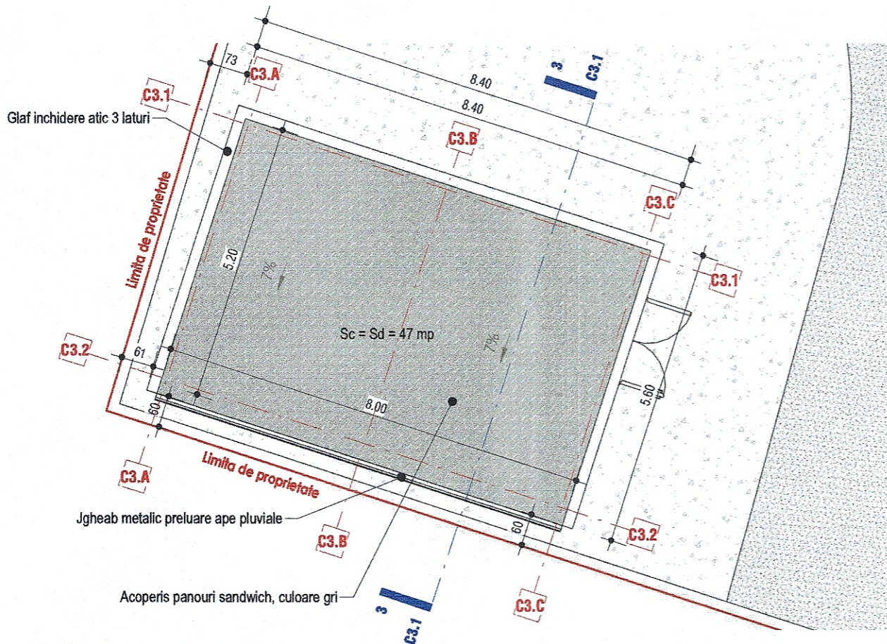
PLAN ACOPERIS - CORP C3 STATIE POMPE
