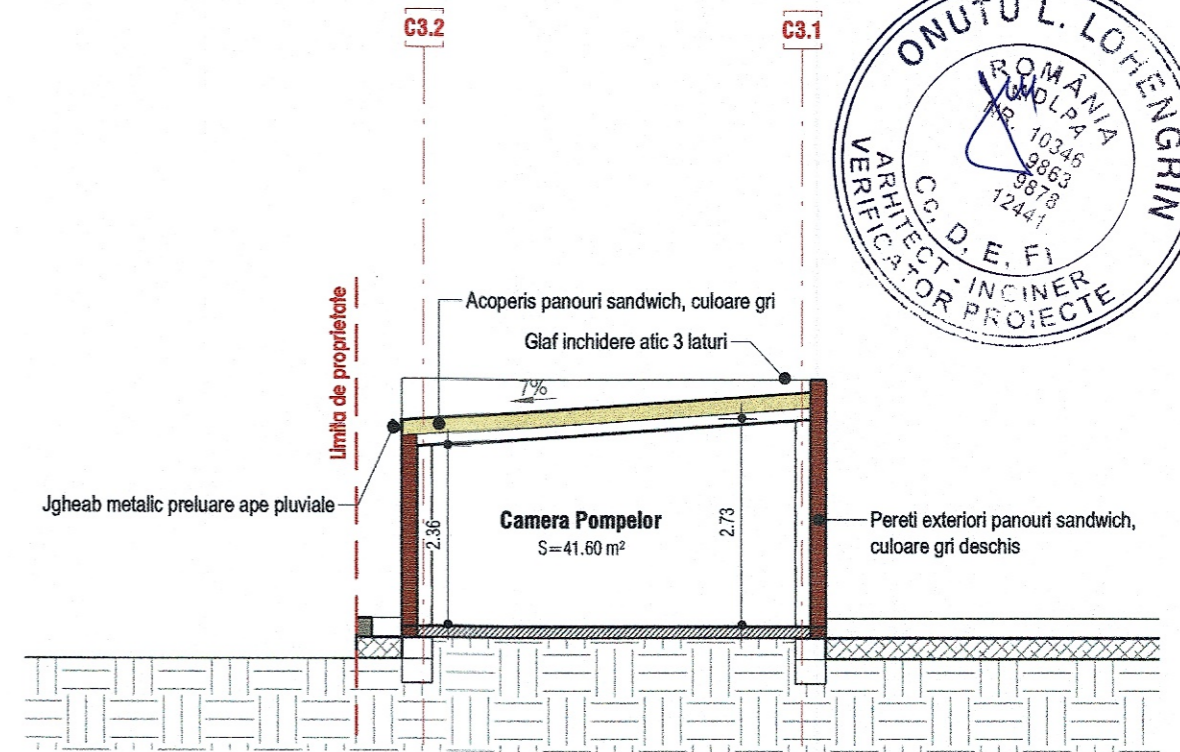
SECTIUNE - CORP C3 STATIE POMPE
