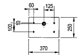
Vedere din fata 1:20
