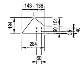
Vedere din fata 1:20
