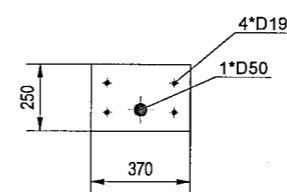
Vedere din spate 1:20
