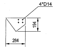
Vedere din spate 1:20
