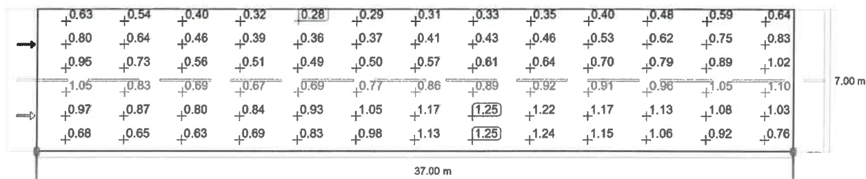
Observator 2: Valoarea de întreținere, densitatea luminii cu carosabil uscat [ \text{cd}/\text{m}^2 ] (Linii Isolux)
